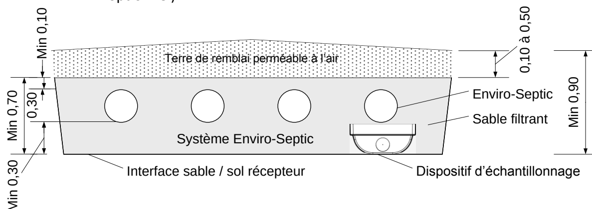
Figure 4 - Vue en coupe d'un Système Enviro-Septic en infiltration
