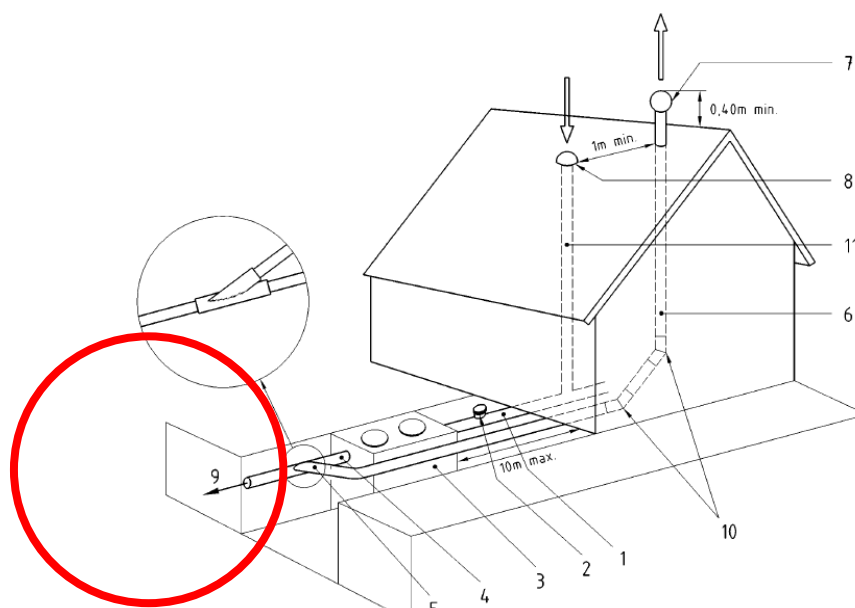
Figure 13 – Schéma de principe – ventilation de la fosse septique
