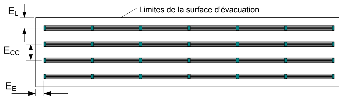
Figure 3 - Espacements des rangées de conduites
